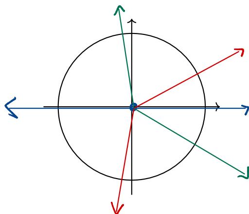
Unit Circle
