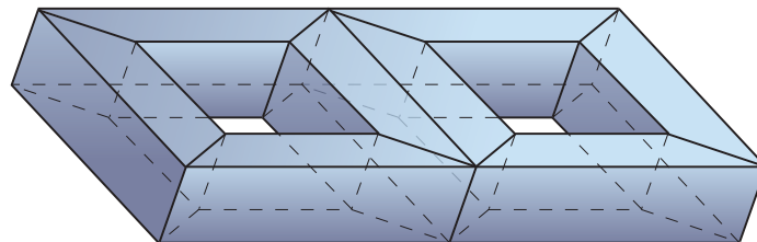
double torus ( g=2 )
