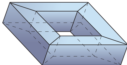
torus ( g=1 )
